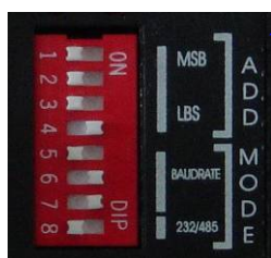
SC600E 面板开关
